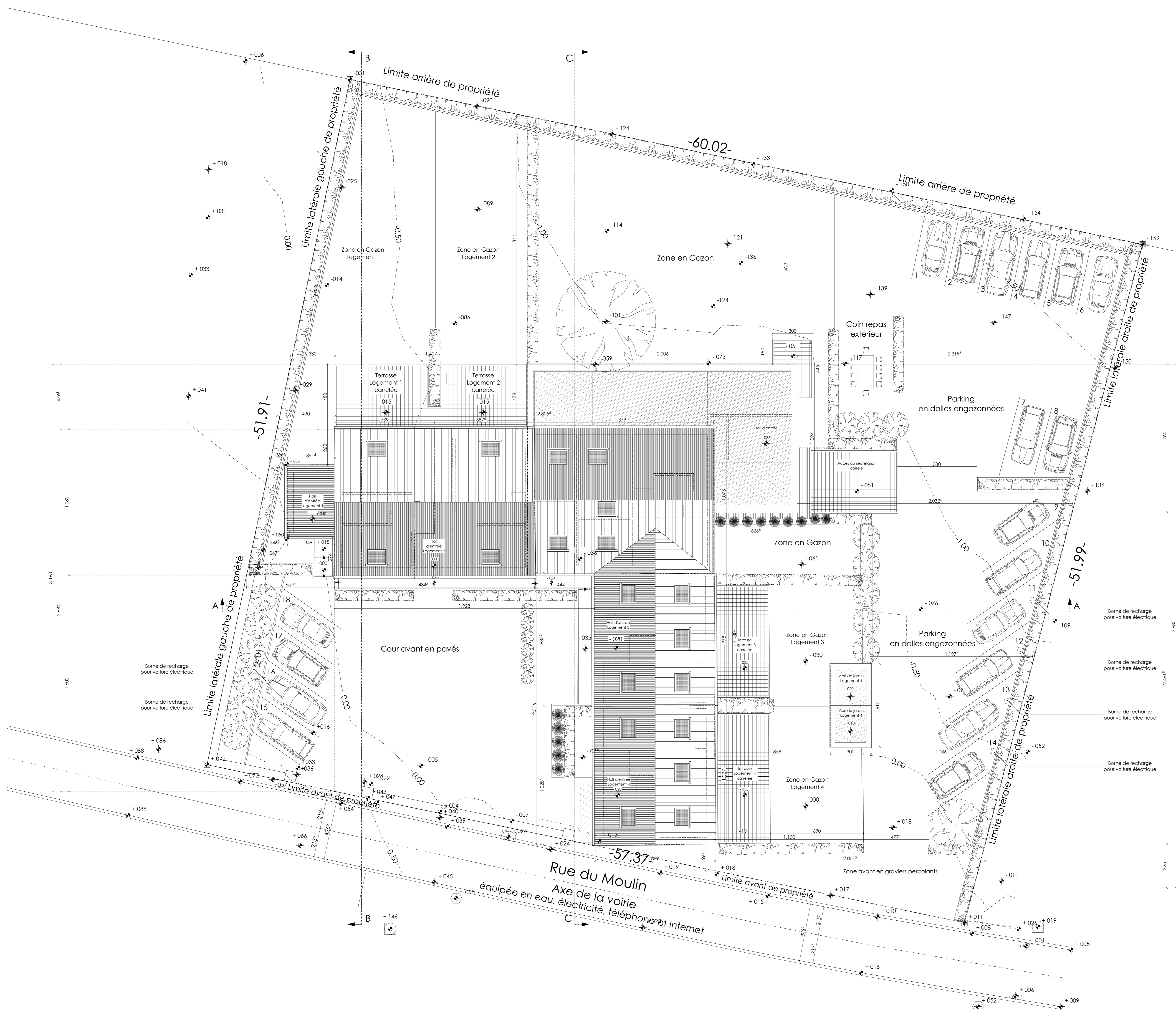
SITUATION PROJETEE - VUE EN PLAN Implantation - Ech.: 1/100
